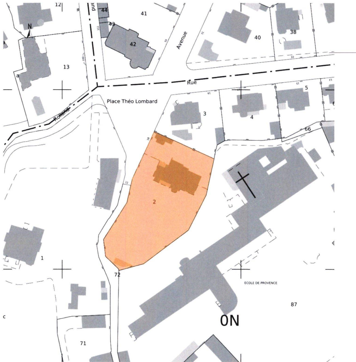
CADASTRE ECH 1/1000E
