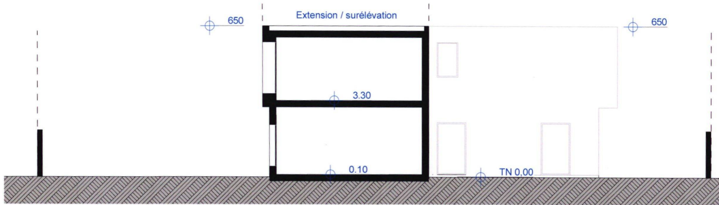
Etat projeté
