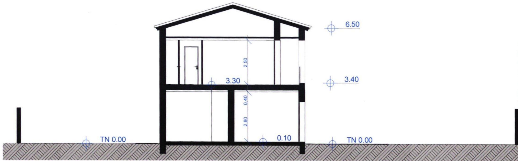
Etat existant
